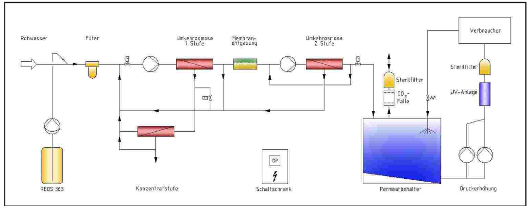
Verfahrensschema einer zweistufigen Umkehrosmose mit Konzentrataufb.
