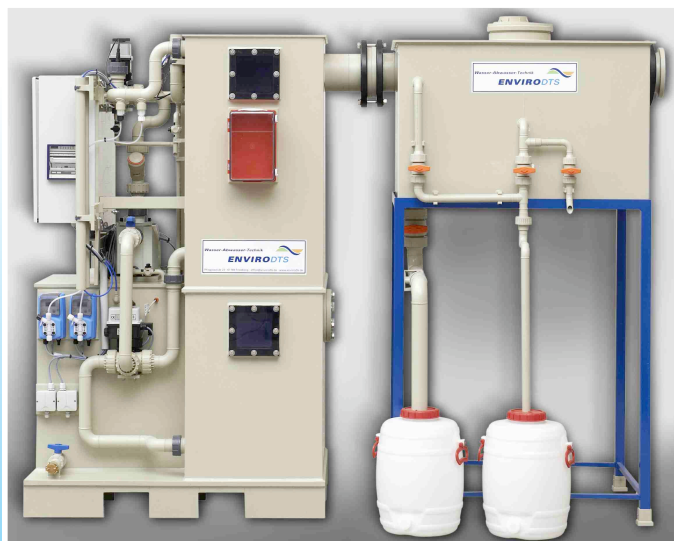
regelbare Dosierpumpen
