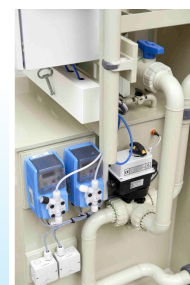
regelbare Dosierpumpen
