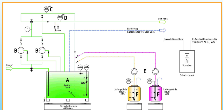
Verfahrensschema der Neutro-Fix 3K
